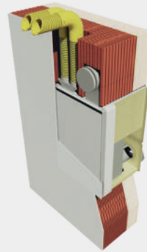
PROVEDENÍ S INTEGRACÍ DO STĚNY U 2 S KANÁLOVOU PŘÍPOJKOU
