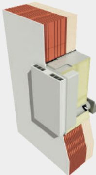
PROVEDENÍ POD OMÍTKU
