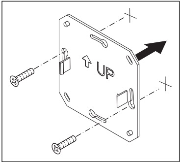
Abb. 3: Montageplatte befestigen
