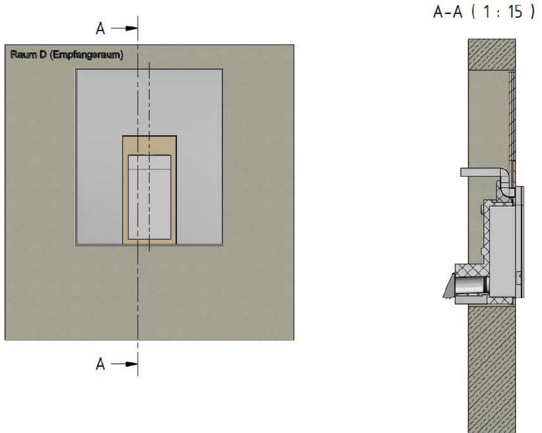
Abbildung F.6. Mehr-Raum-Variante mit Kanalanschluss ABL- und ZUL-seitig: Innenansicht und Vertikalschnitt des Prüfaufbaus.
