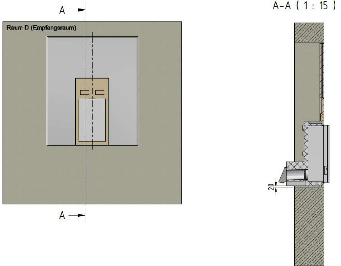
Abbildung F.3. Ein-Raum-Variante: Innenansicht und Vertikalschnitt des Prüfaufbaus.
