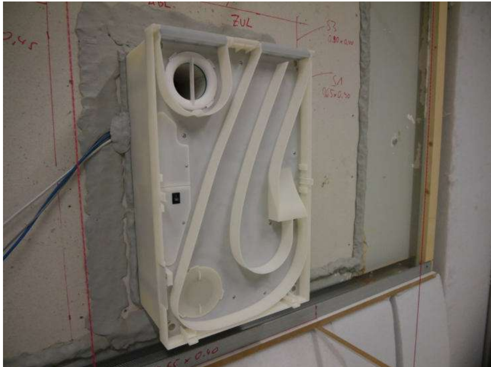
Abbildung B.9. Ansicht Lüftungsgerät innenseitig nach Montage auf der Trockenbaublende im Fensterprüfstand, Gerätedeckel entfernt.
