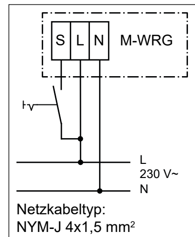
Abb. 12: Anschlussplan für ext. Steuereingang
