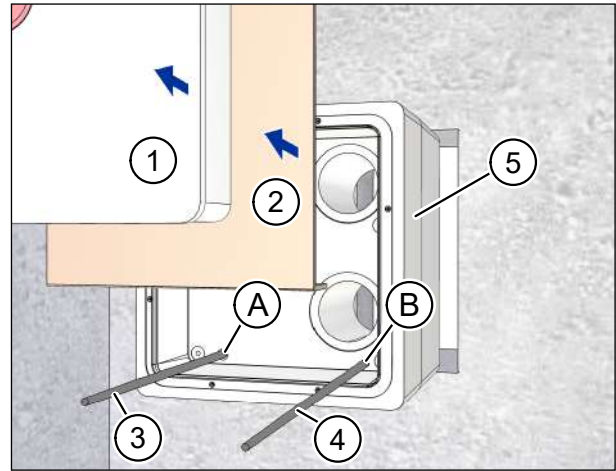
Abb. 13: Mauerkasten einsetzen
