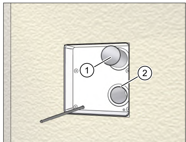
Abb. 28: Lüftungsrohre ablängen
