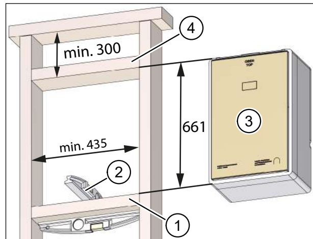
Abb. 45: Aufnahme für Montageset in Ständerkonstruktion erstellen – Maße in Millimeter
