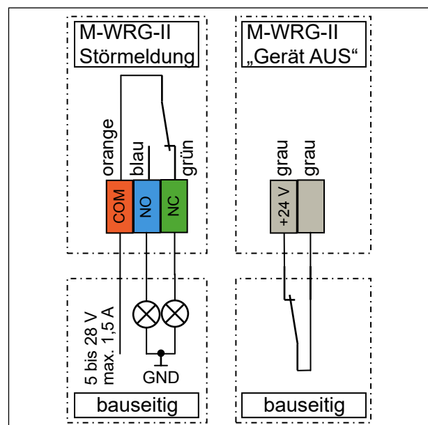
Abb. 21: Anschlusspläne für Option M-WRG-II O/EGG-AUS
