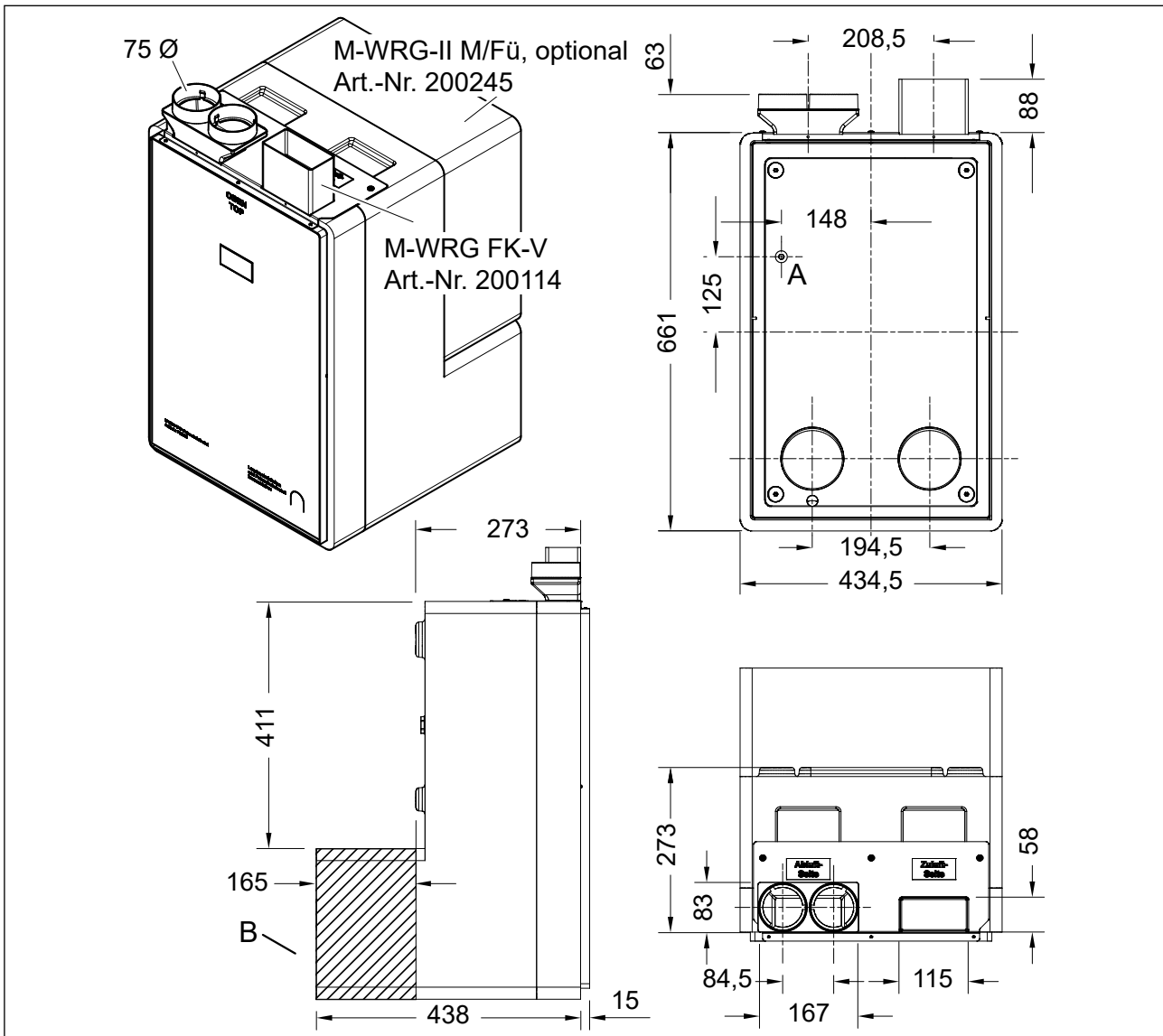
Abb. 8: Abmessungen des Montagesets mit optionalem Füllstück in Millimeter
