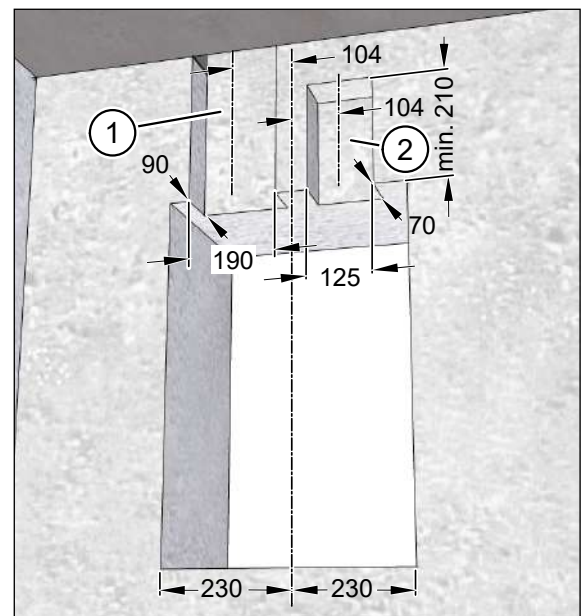
Abb. 16: Mauernuten für Flexrohr- und Flachkanalanschluss fräsen, Maße in Millimeter
