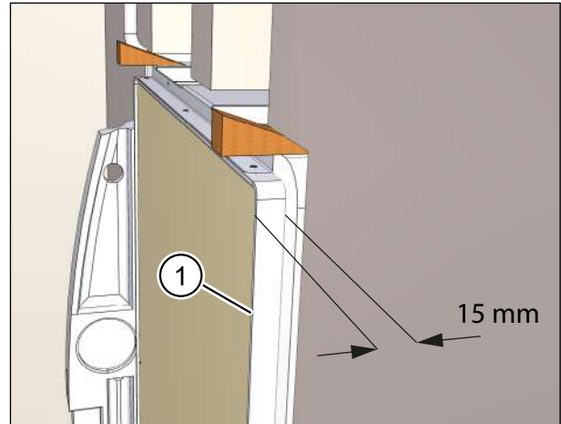
Abb. 25: Putzrahmentiefe 15 mm
