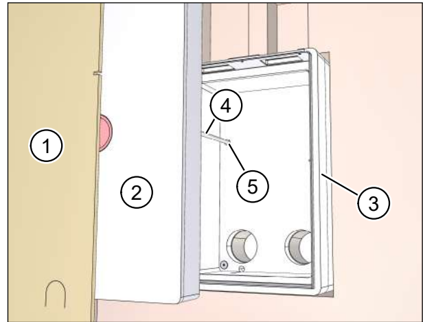
Abb. 22: Mauerkasten einsetzen
