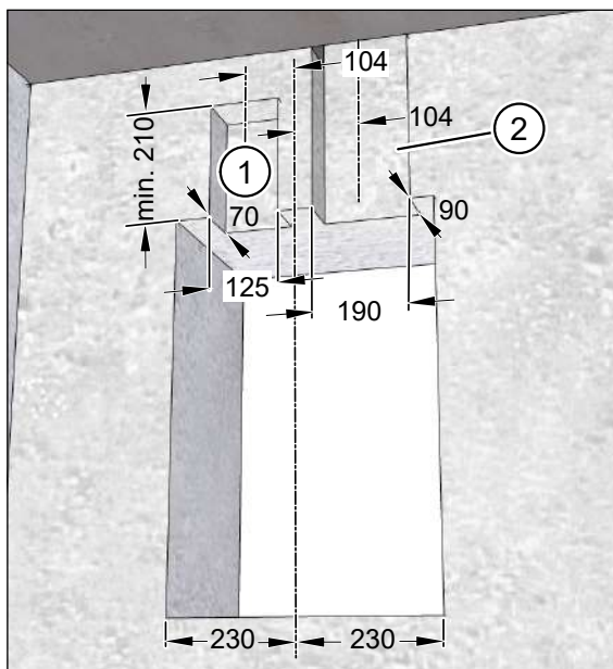
Abb. 15: Mauernuten für Flachkanal- und Flexrohranschluss fräsen, Maße in Millimeter
