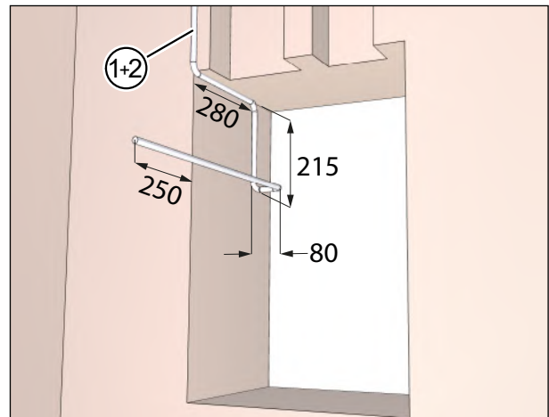
Abb. 19: Anschlusskabel verlegen, Maße in Millimeter
