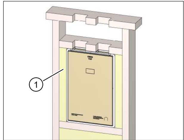
Abb. 54: Hohlräume um den Mauerkasten mit Dämmmaterial füllen
