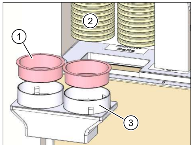
Abb. 57: Flexrohre ablängen
