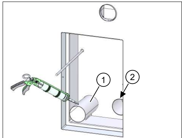
Abb. 42: Lüftungsrohre einsetzen und fixieren
