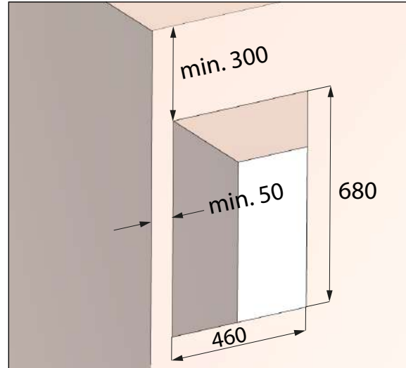
Abb. 10: Mauerdurchbruch für Montageset mit Füllstück, Maße in Millimeter
