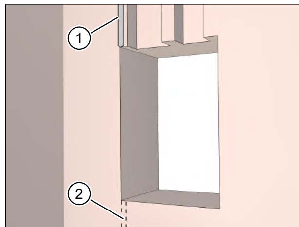
Abb. 18: Mauernuten für Anschlusskabel fräsen
