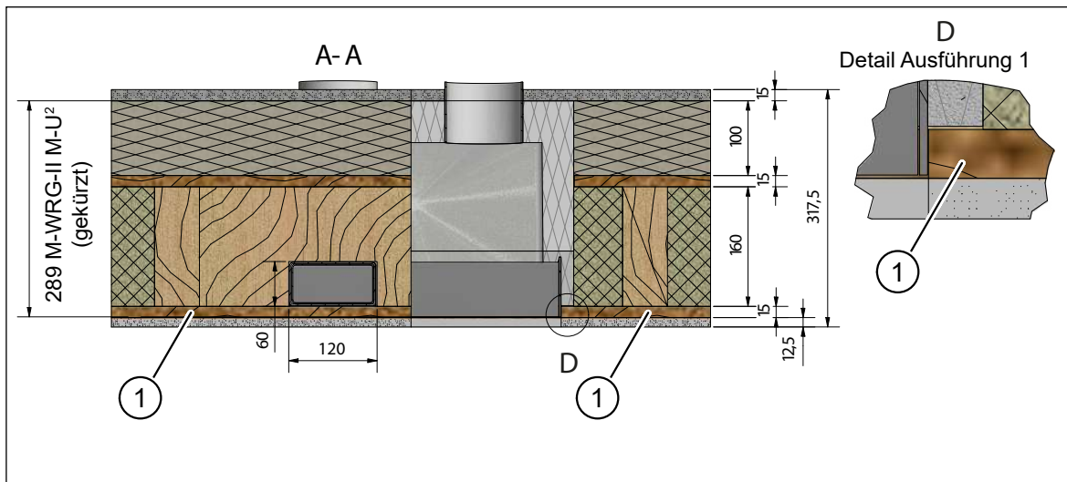
Abb. 55: Innere OSB-Platte als Dampfbremse und luftdichte Ebene
