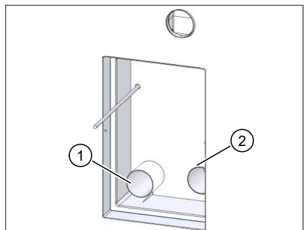
Abb. 41: Lüftungsrohre ablängen
