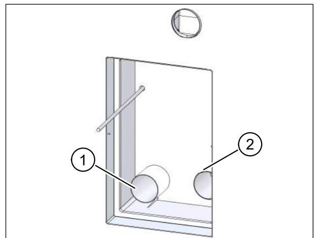
Abb. 70: Lüftungsrohre ablängen
