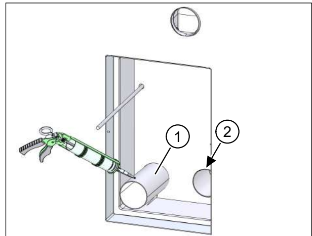
Abb. 71: Lüftungsrohre einsetzen und fixieren
