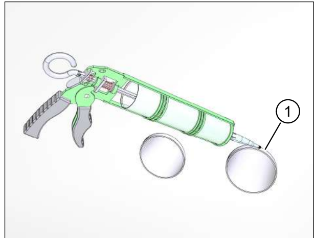
Abb. 72: Lüftungsrohre an der Außenwand abdichten
