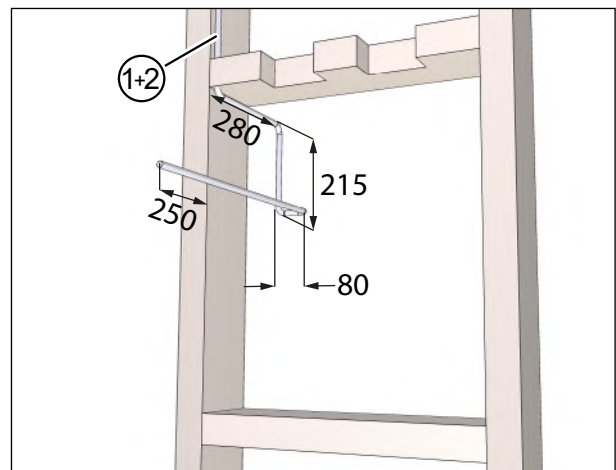
Abb. 47: Anschlusskabel verlegen, Maße in Millimeter
