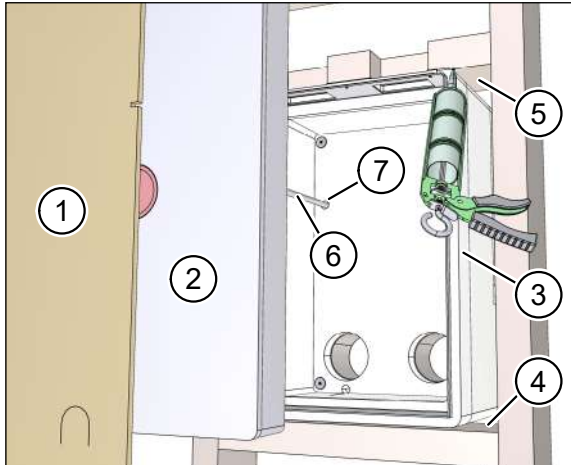
Abb. 50: Mauerkasten einsetzen und fixieren
