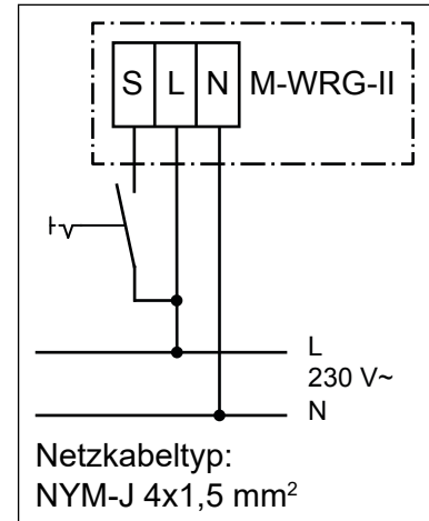
Abb. 48: Anschlussplan für ext. Steuereingang
