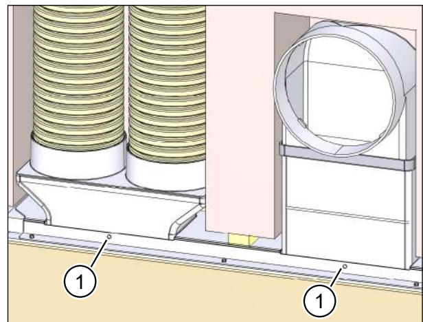
Abb. 59: Flachkanal- / Flexrohranschlüsse am Mauerkasten befestigen
