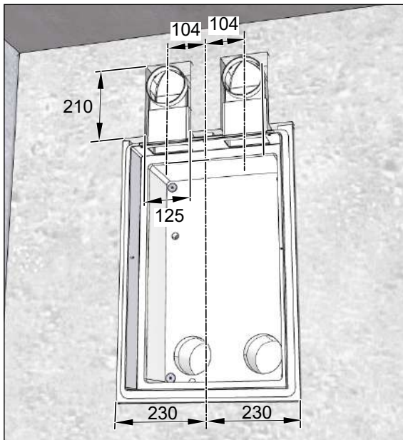
Abb. 12: Beispiel für vertikale Flachkanalführung, Maße in Millimeter
