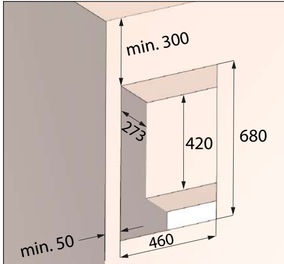
Abb. 9: Mauerdurchbruch für Montageset ohne Füllstück, Maße in Millimeter
