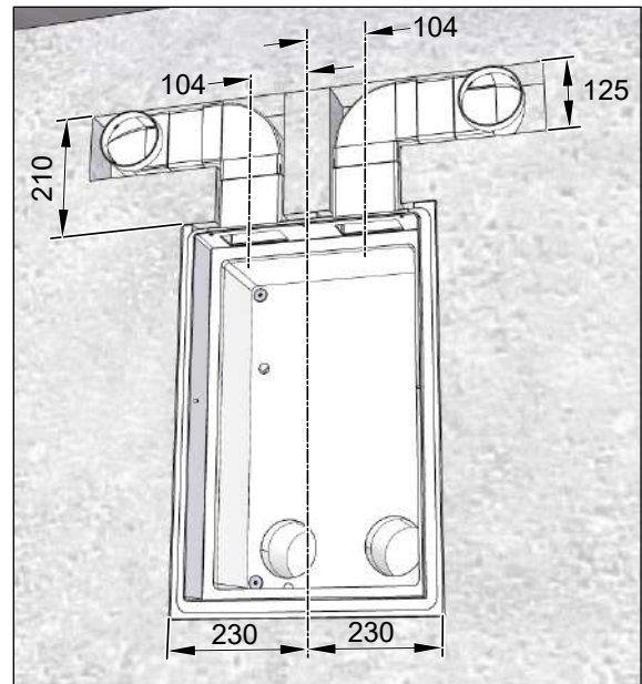
Abb. 13: Beispiel für horizontale Flachkanalführung, Maße in Millimeter
