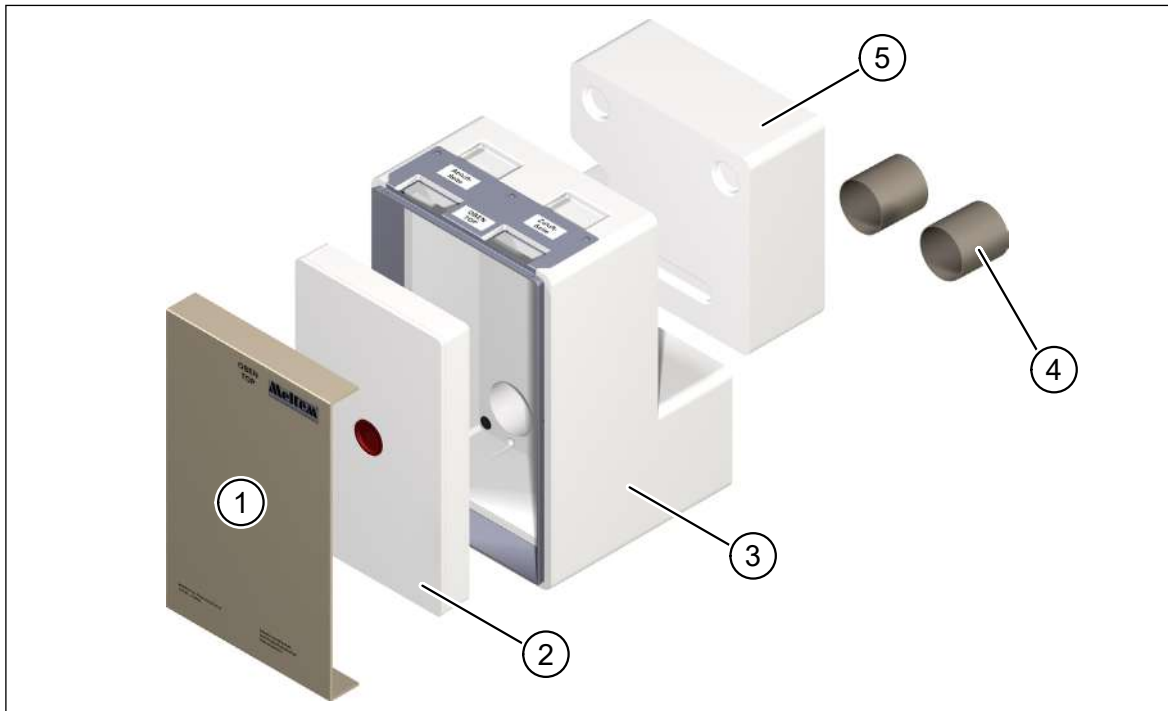
Abb. 7: Lieferumfang Montageset M-WRG-II M-U 2
