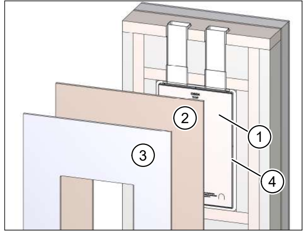
Abb. 60: Montageset und Flachkanäle / Flexrohre im Innenbereich verkleiden
