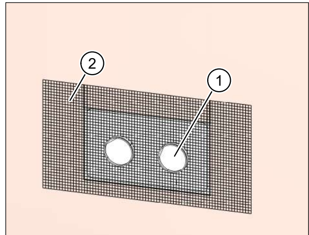
Abb. 66: Montageset ohne Füllstück einputzen
