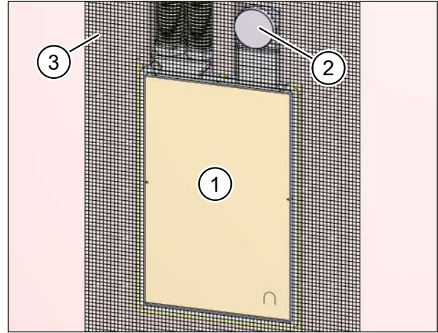
Abb. 31: Montageset und Flachkanäle / Flexrohre im Innenbereich einputzen
