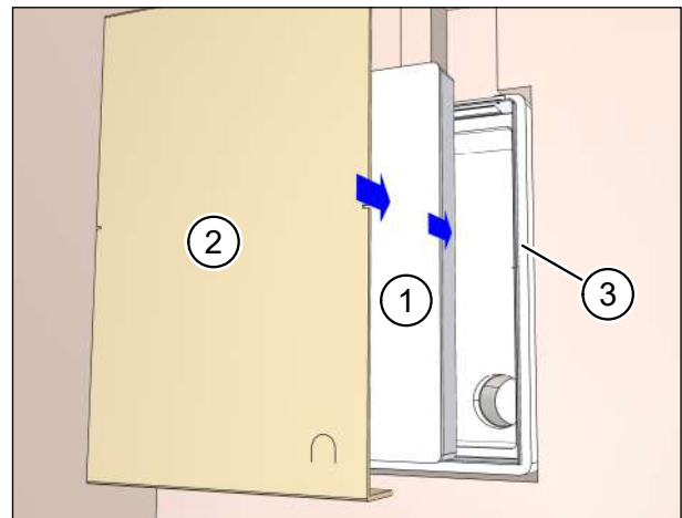
Abb. 23: Schutzdeckel und Putzschutzdeckel einsetzen
