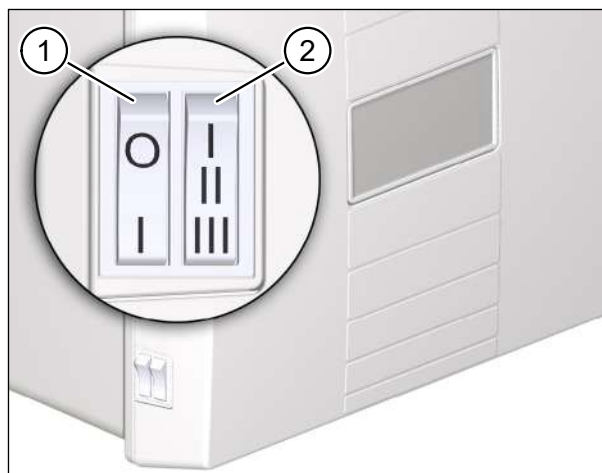
Abb. 11: Bedienungselemente am Lüftungsgerät
