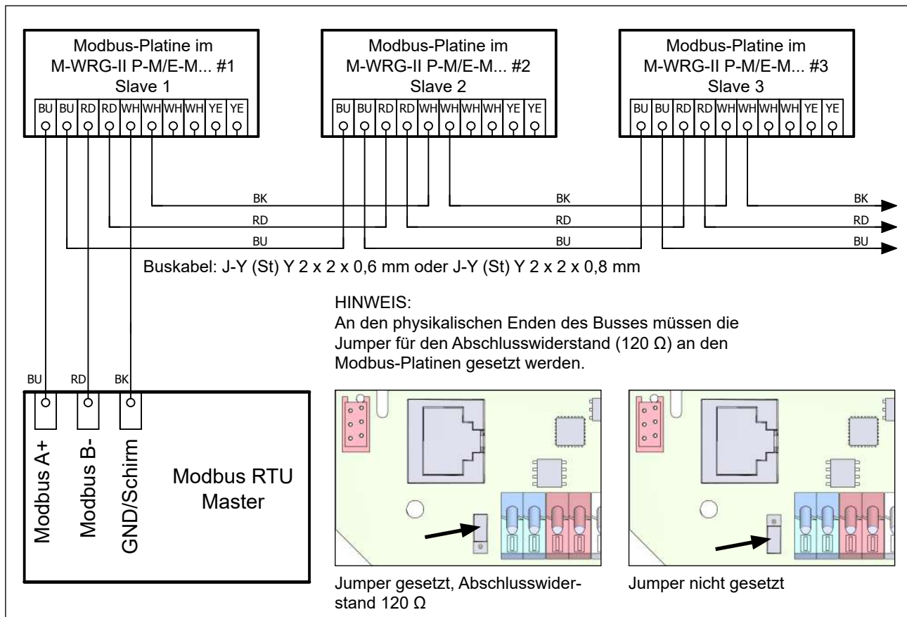
Abb. 24: Anschlussschema Modbus
