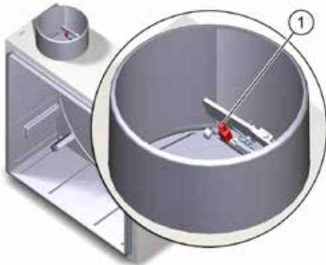
Abb. 5: Gehäusetyp UBK
